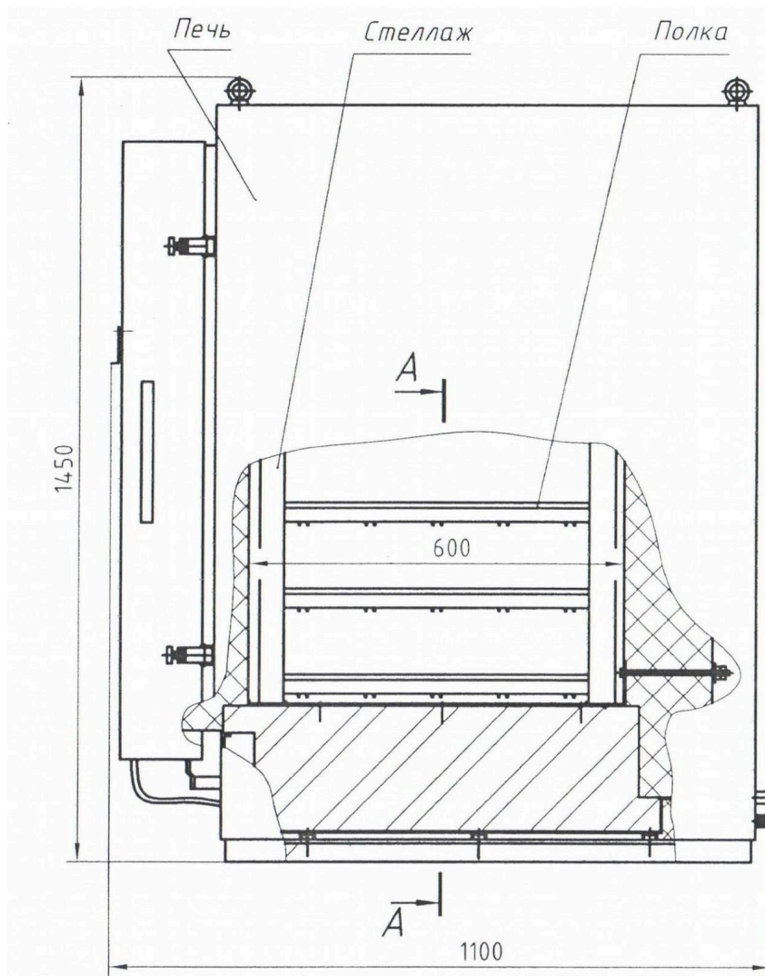
Рис.2.1. Общий вид печи со стеллажом.
