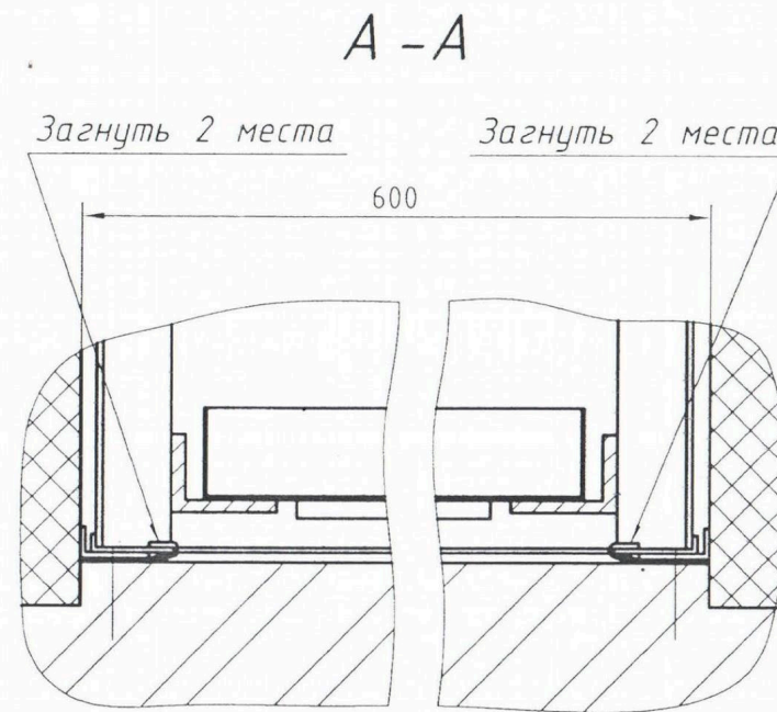
Рис.2.2. Монтаж стеллажа в камере печи.
